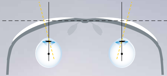
► Sportbrille mit stark verkippten Gläsern Augendrehtpunktforderung wird nicht erfüllt
